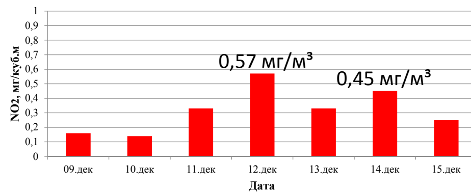
г. Иркутск (ул. Сухэ-Батора), содержание в воздухе NO 2
