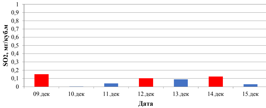
г. Иркутск (ул. Севастопольская), содержание в воздухе SO 2
