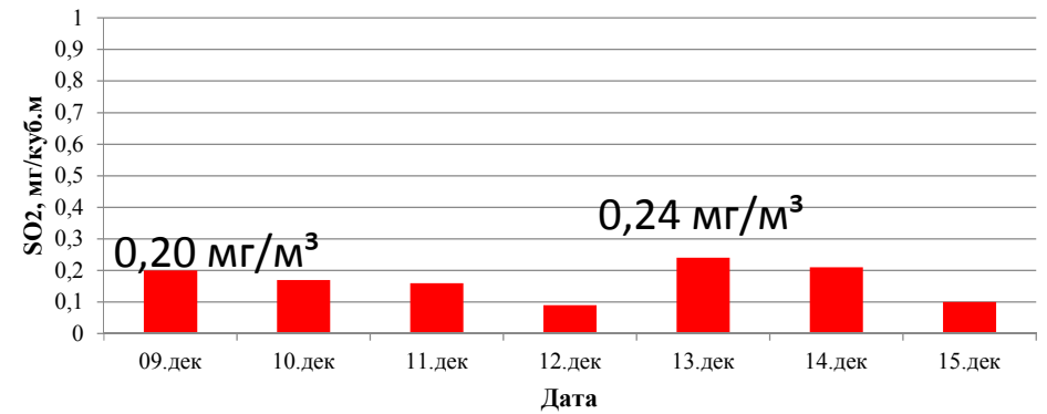
г. Иркутск (ул. Сухэ-Батора), содержание в воздухе SO 2
