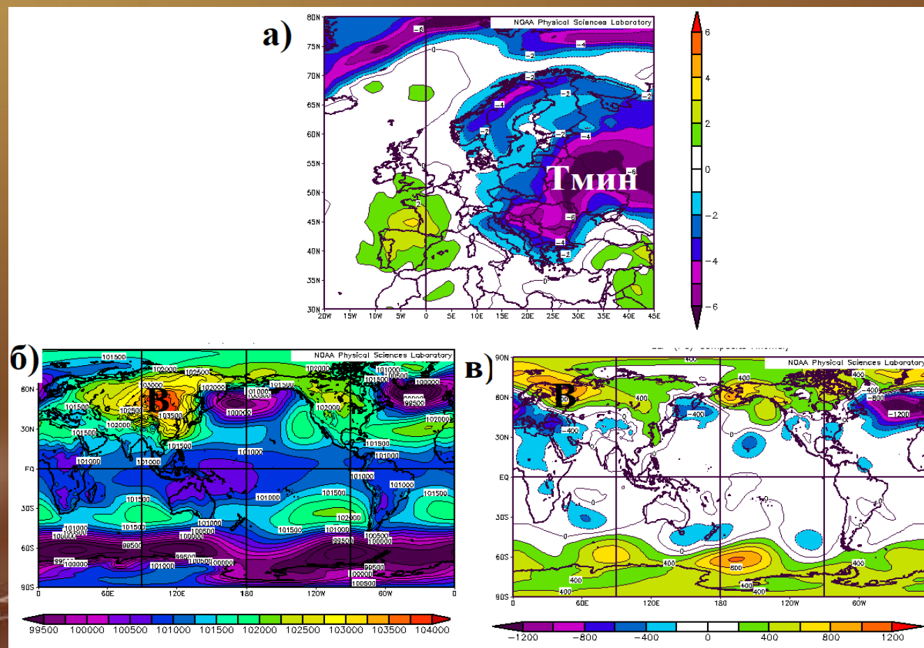
Карты аномалий минимальной температуры воздуха (а), среднего поля атмосферного давления у поверхности Земли (б) и его аномалий (в) в январе 1943 г
