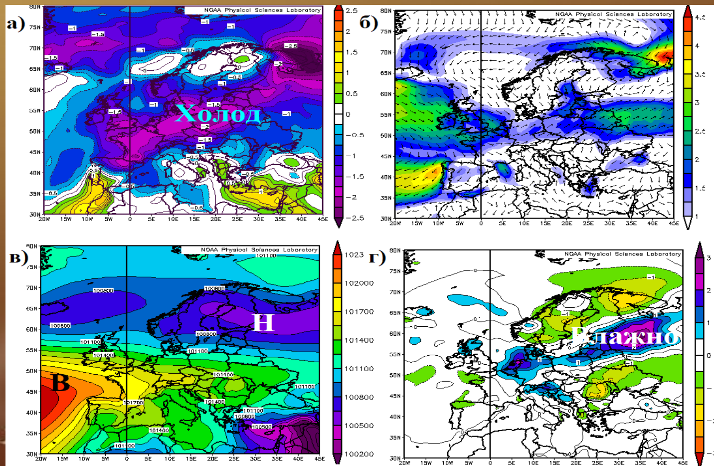
Карты аномалий приземной температуры воздуха (а), потоков ветра (б), атмосферного давления (в) и атмосферных осадков (г) у поверхности Земли в июле 1942 г
