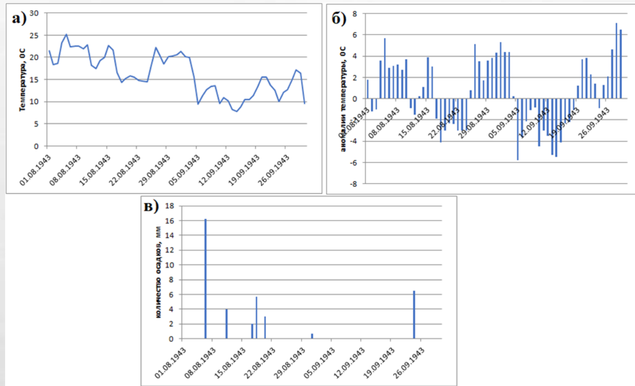
ИЗМЕНЕНИЕ СРЕДНЕЙ СУТОЧНОЙ ТЕМПЕРАТУРЫ ВОЗДУХА (А), АНОМАЛИЙ ТЕМПЕРАТУР (Б) И СУММ АТМОСФЕРНЫХ ОСАДКОВ В ПЕРИОД ПРОВЕДЕНИЯ ДОНБАССКОЙ ОПЕРАЦИИ В 1943 ГОДУ
