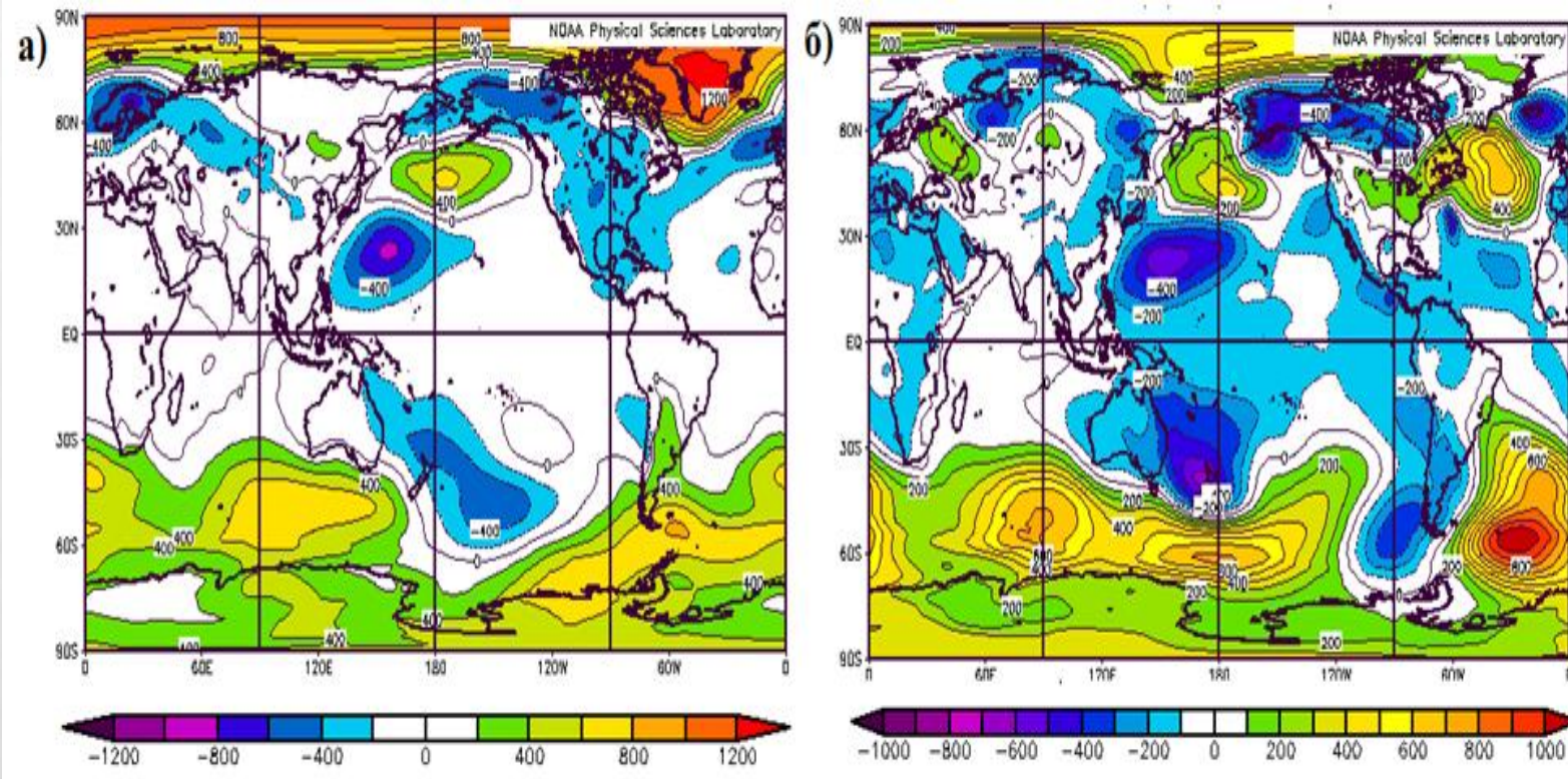
2 КАРТЫ АНОМАЛИЙ ПРИЗЕМНОГО ДАВЛЕНИЯ В АВГУСТЕ (А) И СЕНТЯБРЕ (Б) 1943 Г.
